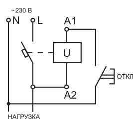
Схема подключения
